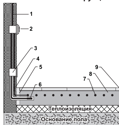
Конструкция пола с подогревом
