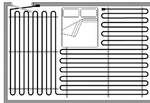
Конструкция пола с подогревом
