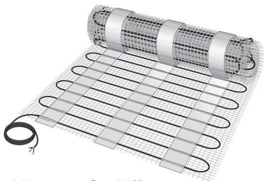
1. Нагревательный мат W160 с проводом для подключения длиной 2 м.
